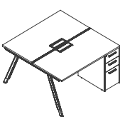
DN61 W1200•D1228•H750(mm) W1400•D1428•H750(mm) W1500•D1428•H750(mm) W1600•D1428•H750(mm)
