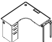
DN62AL/R W1428•D1428•H750(mm) W1528•D1528•H750(mm) W1628•D1628•H750(mm)
