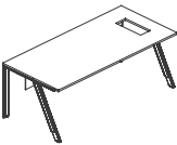
DN85 W1600•D750•H750(mm) W1800•D900•H750(mm) W2000•D900•H750(mm)
