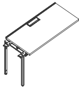
DN60A W1200•D628•H750(mm) W1400•D728•H750(mm) W1500•D728•H750(mm) W1600•D728•H750(mm)
