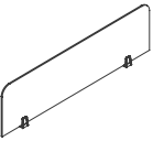
DNBP W530•350•H32(mm) W880•350•H32(mm) W1080•350•H32(mm) W1180•350•H32(mm) W1280•350•H32(mm) W1380•350•H32(mm) W1480•350•H32(mm) W1580•350•H32(mm)
