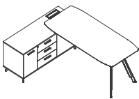
DN88L/R W2250•D1780•H750(mm) W2450•D1780•H750(mm)
